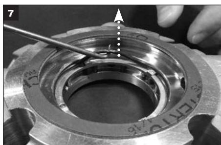
Poista O-rennas (X) laipan O-renkaan urasta ja hävitä.
