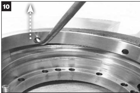
Tiivisteet, joissa on injektorilisävaruste: Irrota injektori varovasti ja aseta se sivuun.
