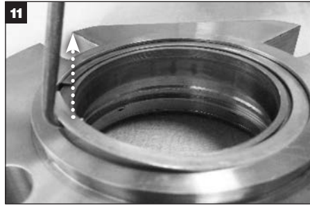
Tiivisteet, joissa on holkkisarja: Irrota joustorengas laipasta ja hävitä se.
