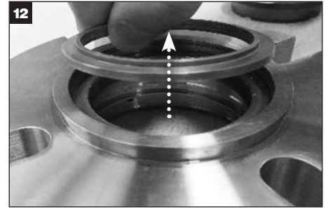
Tiivisteet, joissa on holkkisarja: Irrota holkki ja holkin O-rengas (Y) laipan reiästä ja hävitä ne.
