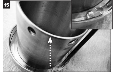
Irrota asetusputki holkissa olevista asetuskorvakkeista ja hävitä se.
