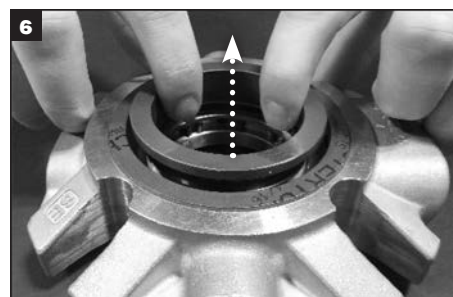
Irrota kiinteä tiivisterengas laipasta ja hävitä se.
