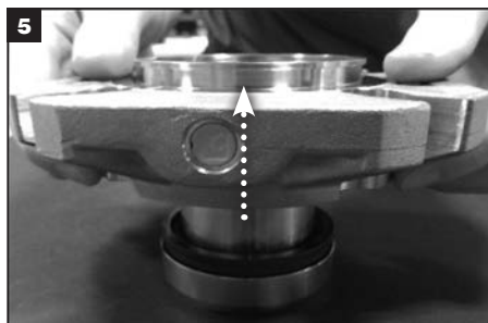
5 グランドからスリーブを分離し、スリーブを脇に置きます。
