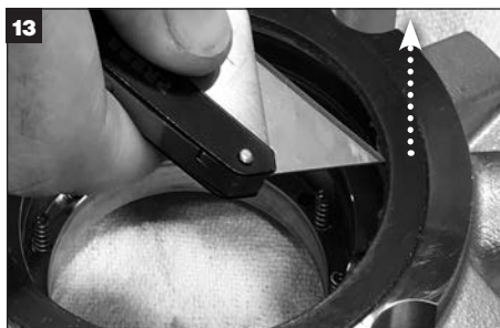
グランドからスタフリングボックスフェースガasketを外し、廃棄します。
