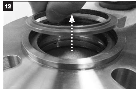
ブッシングキット付きのシール：グランドボアからブッシングとブッシングO-リング (Y)を外し、廃棄します。
