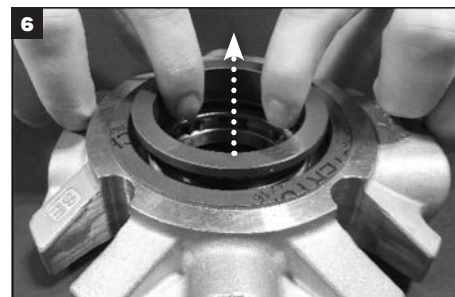
6 グランドから固定環を外し、廃棄します。
