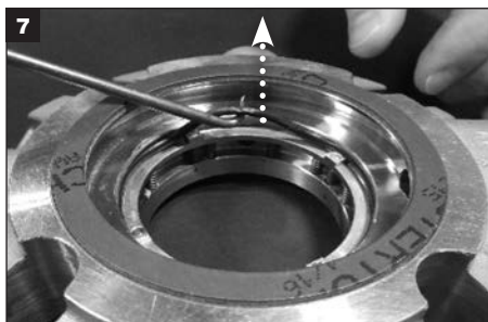
7 グランドO-リングの溝からO-リング(X)を外し、廃棄します。
