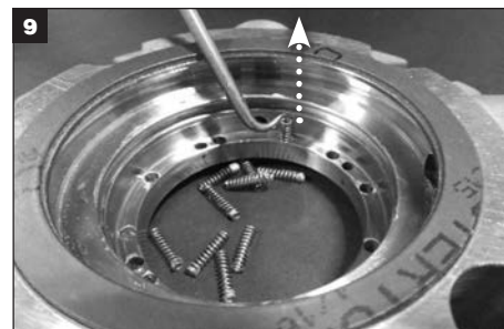
9 グランドスプリングの穴からスプリングをすべて外し、廃棄します。
