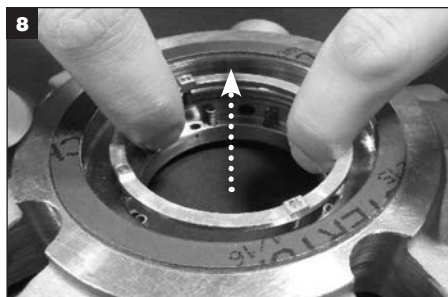
8 グランドからフォロワーアセンブリを外し、脇に置きます。
